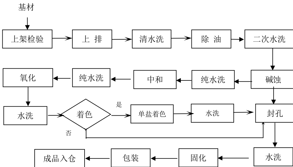
图 2 基材生产工艺流程图
