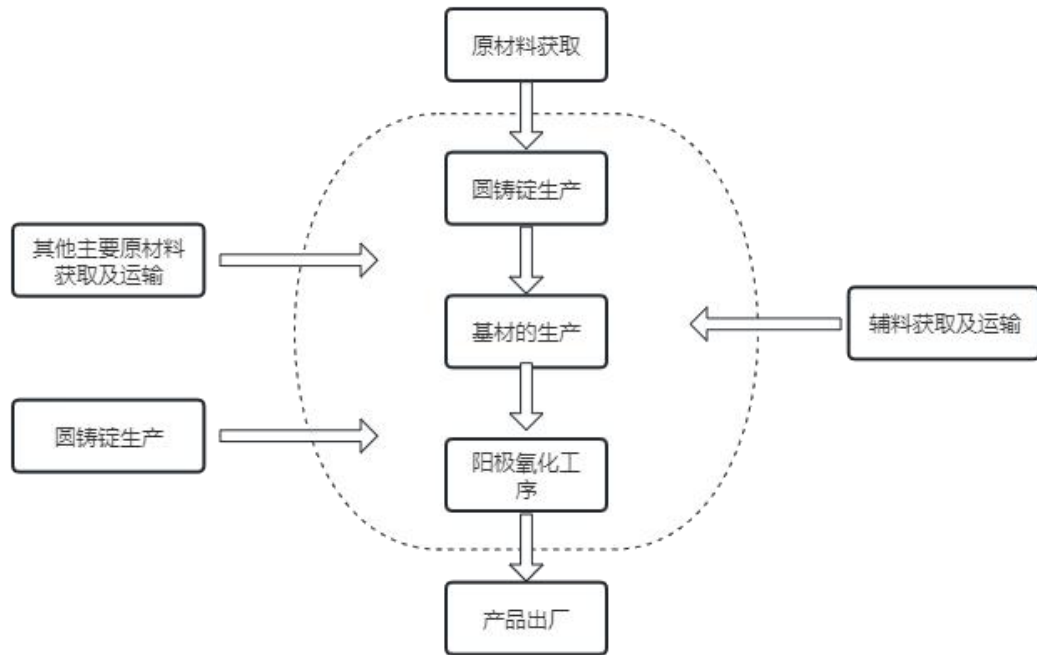
图 3 1t 铝合金建筑型材（阳极氧化型材）产品生命周期系统示意图
