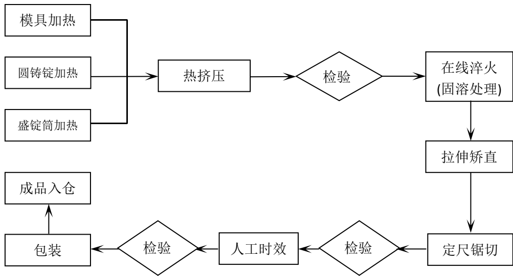
图 2 基材生产工艺流程图
