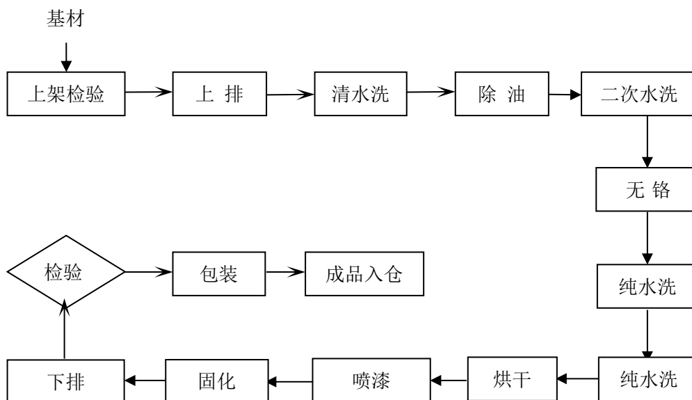
图 3 喷漆工艺流程图
