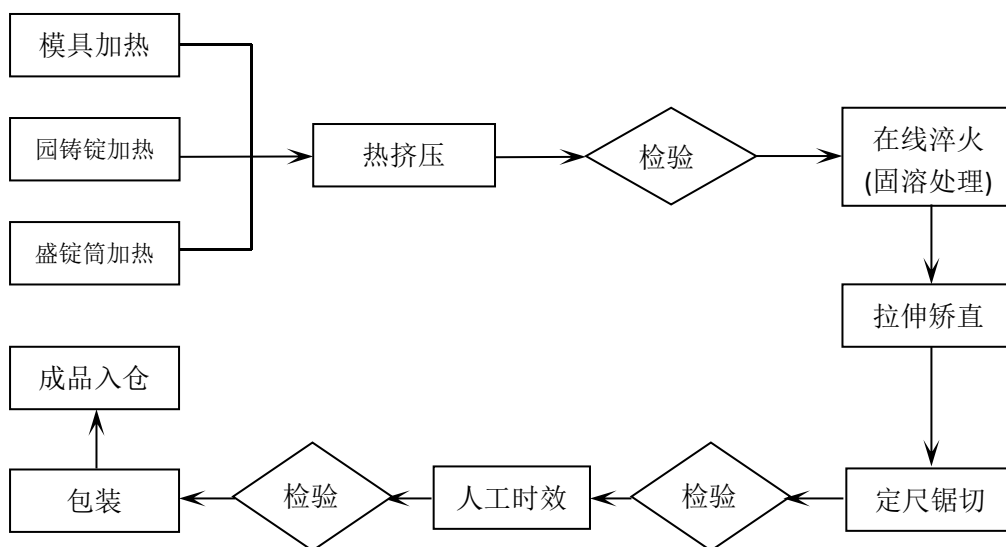
图 2 基材生产工艺流程图
