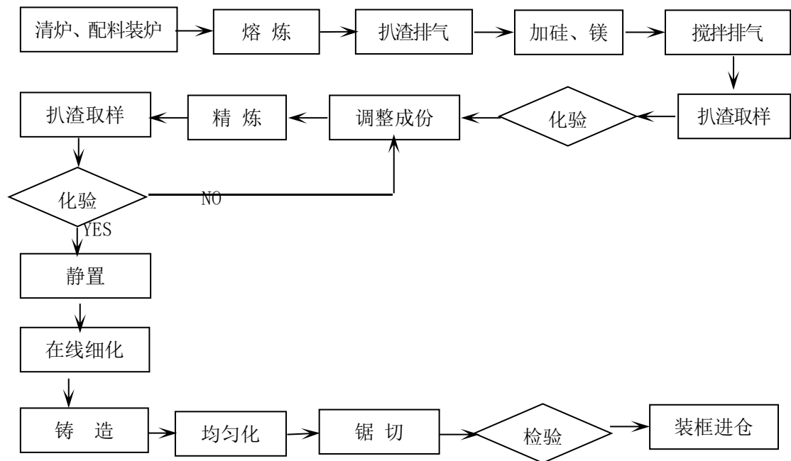
图 1 圆铸锭生产工艺流程图
