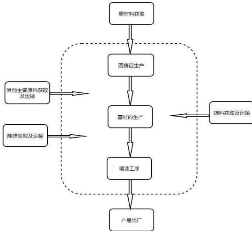
图3 1t 铝合金建筑型材（喷漆型材）产品生命周期系统示意图
