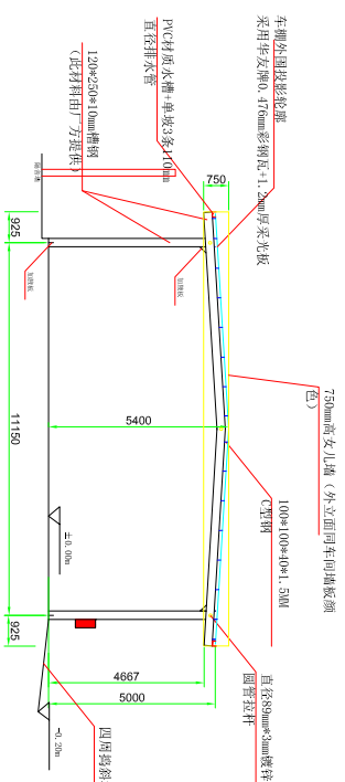
车棚1-1剖面图
